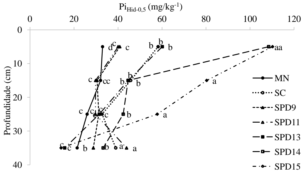
Fig. 16. Fósforo não lábil inorgânico extraído por NaOH 0,5 mol L -1 ( P_{iHid-0,5} ) nas diferentes profundidades e sistemas de manejo do solo em Paragominas, PA. Médias seguidas de mesma letra não diferem entre si pelo teste de Scott-Knott ( p < 0,05 ).
