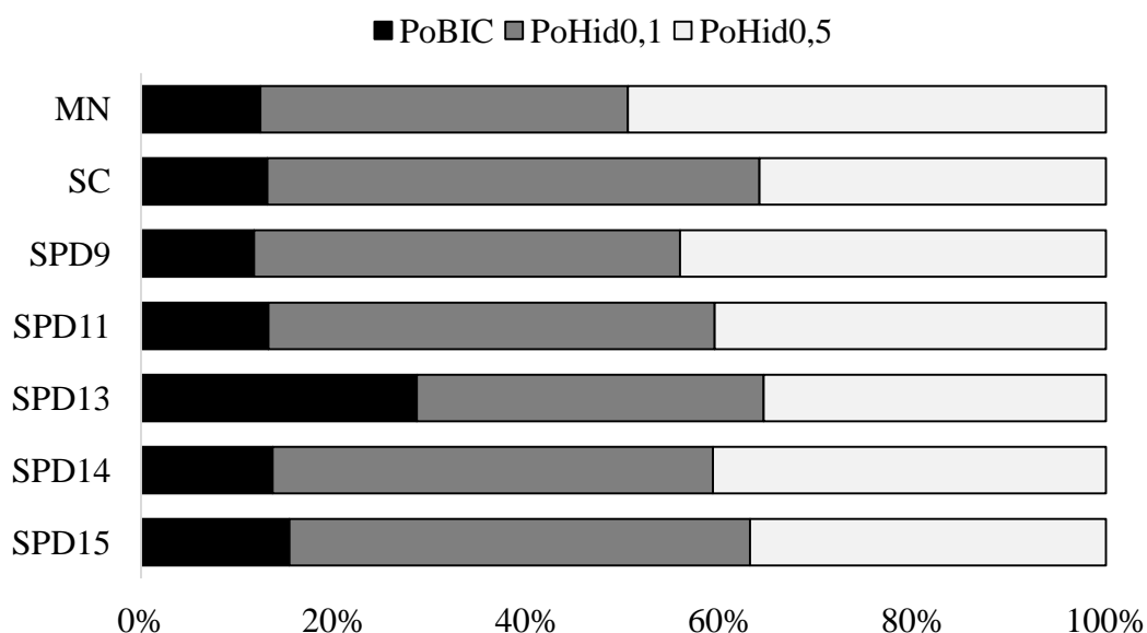
Fig. 22. Distribuição percentual (%) das frações P_{\text{BIC}} , P_{\text{Hid}0,1} e P_{\text{Hid}0,5} no conteúdo de Po-Total em um Latossolo Amarelo distrófico sob diferentes sistemas de manejo em Paragominas, PA.
