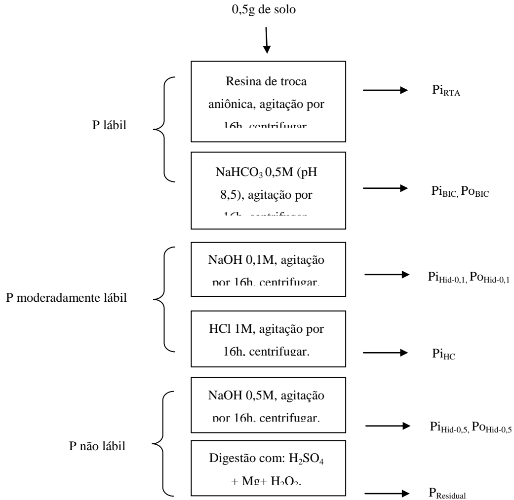
Fig. 3. Diagrama da extração sequencial de fósforo de Hedley et al., (1982), modificado por Condon et al. (1985).
