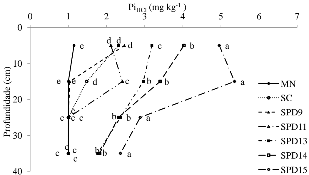
Fig. 14. Fósforo moderadamente lábil extraído por HCl 1 mol L -1 nas diferentes profundidades e sistemas de manejo do solo em Paragominas, PA. Médias seguidas de mesma letra, dentro de cada profundidade, não diferem entre si pelo teste de Scott-Knott ( p < 0,05 ).
