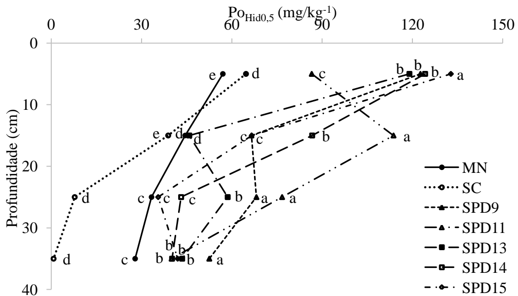
Fig. 17. Fósforo não lábil orgânico extraído por NaOH 0,5 mol L -1 ( P_{oHid0,5} ) nas diferentes profundidades e sistemas de manejo do solo em Paragominas, PA. Médias seguidas de mesma letra, dentro de cada profundidade, não diferem entre si pelo teste de Scott-Knott ( p < 0,05 ).
