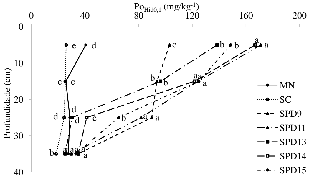
Fig. 13. Fósforo moderadamente lábil orgânico extraído por NaOH 0,1 mol L -1 nas diferentes profundidades e sistemas de manejo do solo em Paragominas, PA. Médias seguidas de mesma letra, dentro de cada profundidade, não diferem entre si pelo teste de Scott-Knott ( p < 0,05 ).
